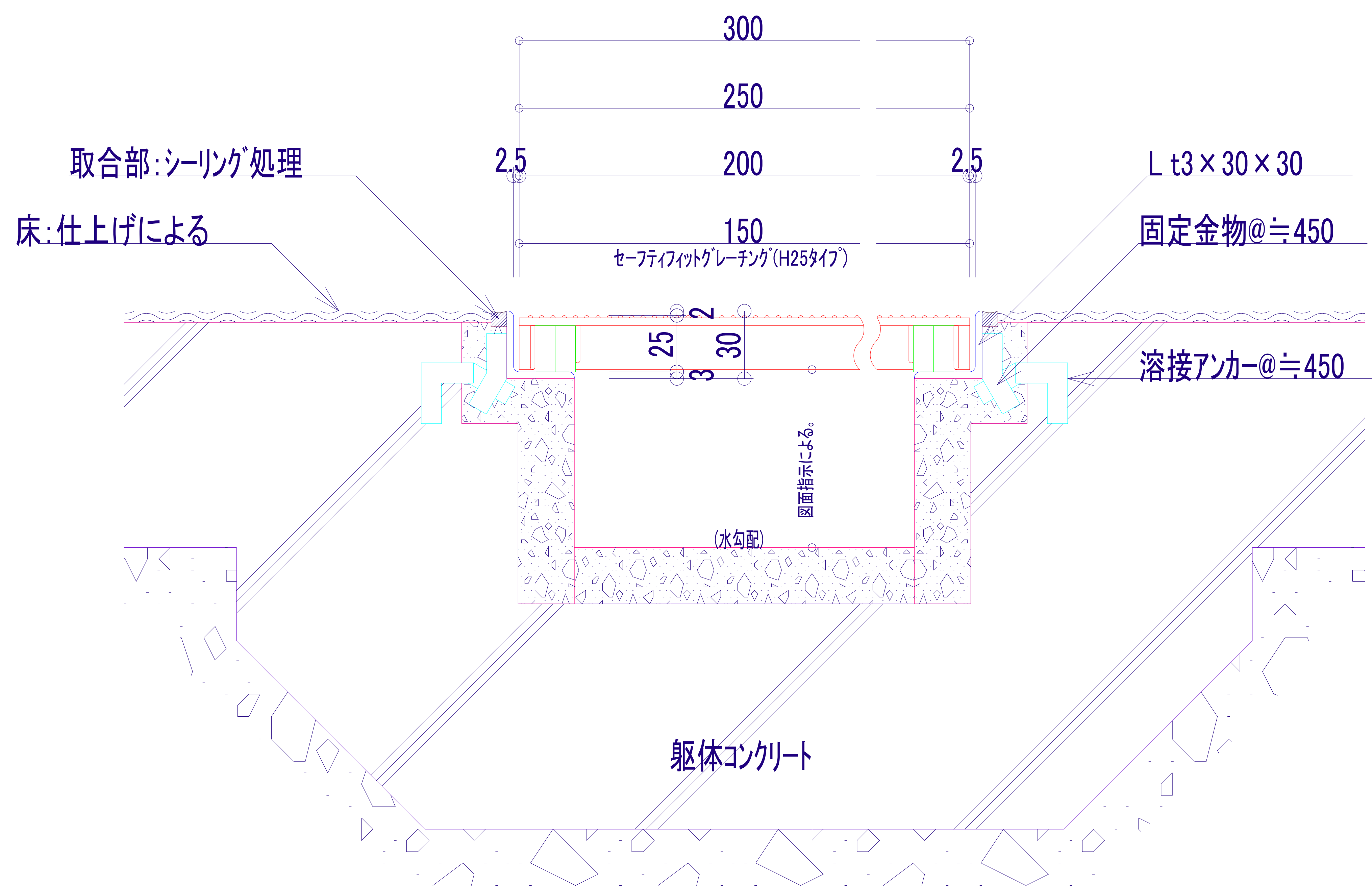
H25タイプ 標準断面図
