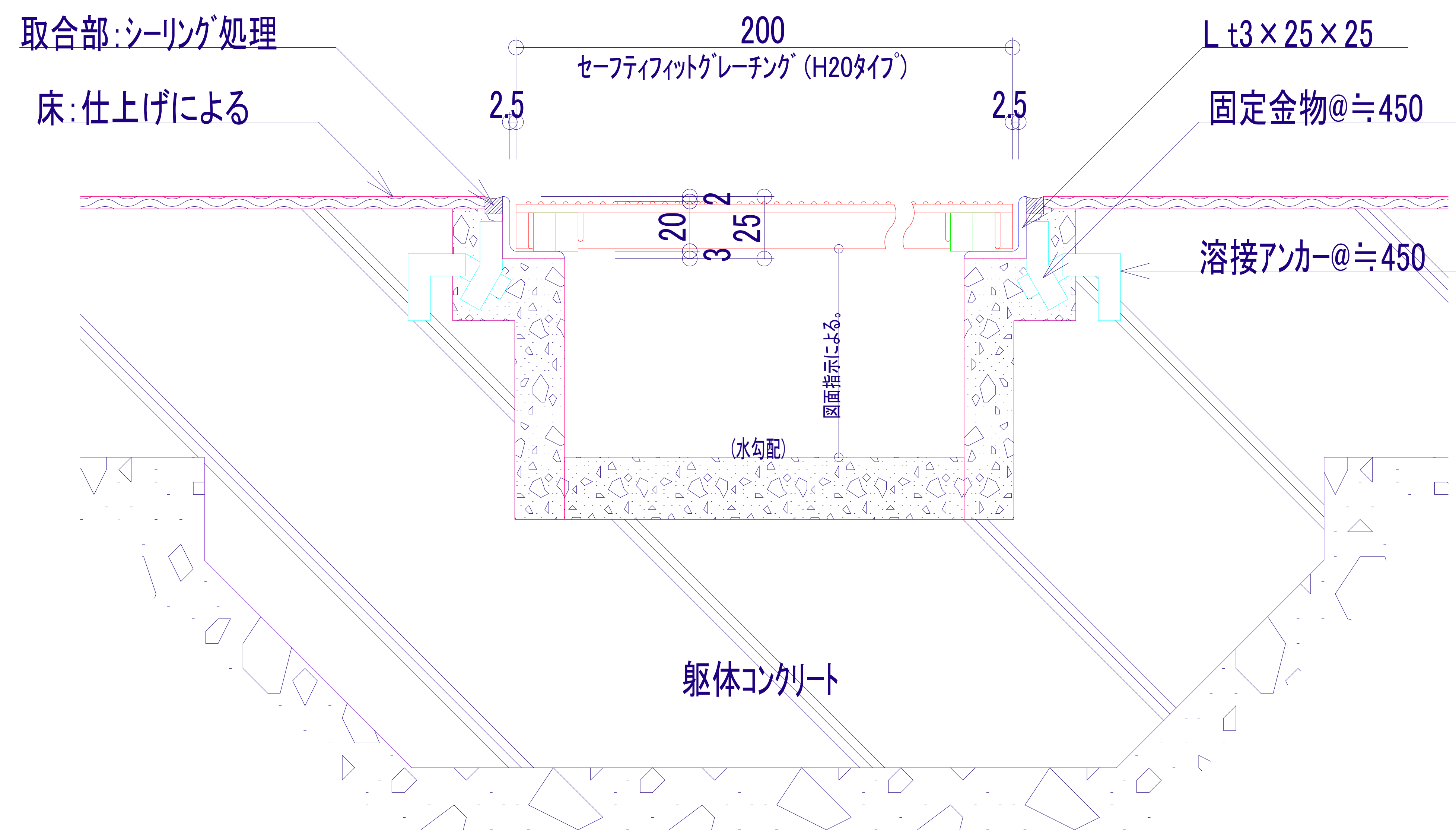
H20タイプ 標準断面図
