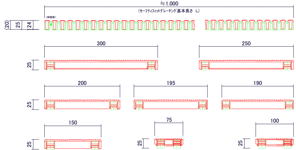
H25タイプ 規格寸法断面図
