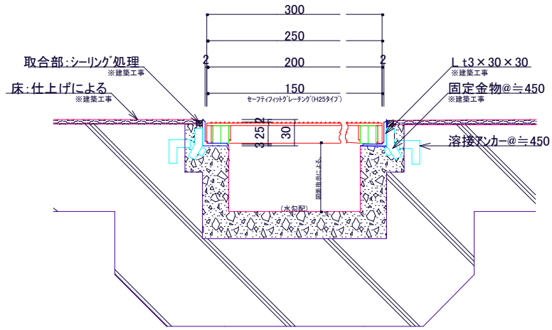
H25タイプ 標準断面図
