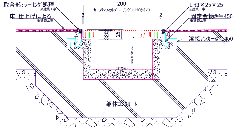
H20タイプ 標準断面図
